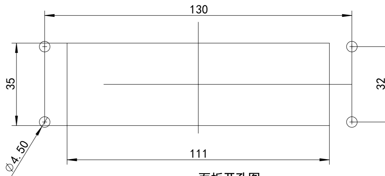
面板开孔图
